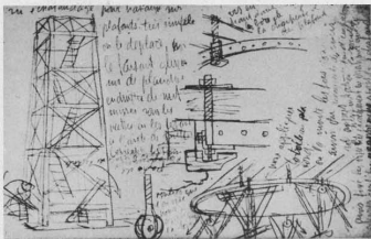
22. Rivera, esbozo de un andamio para trabajo mural en el techo, Italia, 1921. Colección de Jean Charlot.
